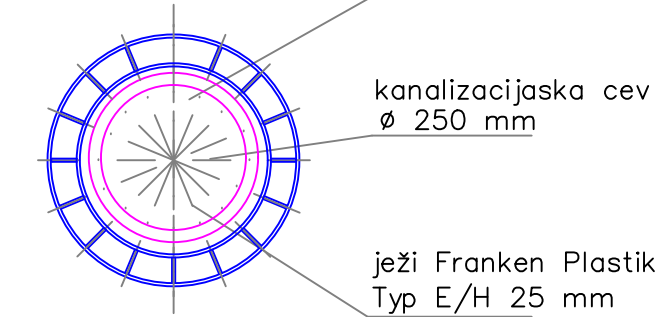
DETALJ ZAŠČITNE CEVI M=1:25
